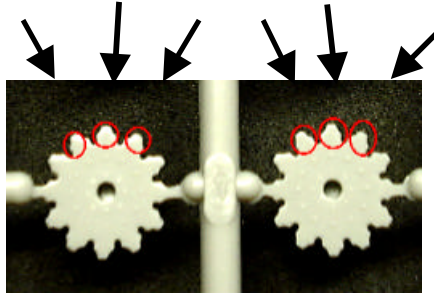
図 8 車体にハセガワキットのスプロケット(部品 # 6、7)を取り付けます。スプロケットのパーツ (部品 # 7) は履帯との干渉を避けるために「歯」を3本削り取ります。(矢印部)
